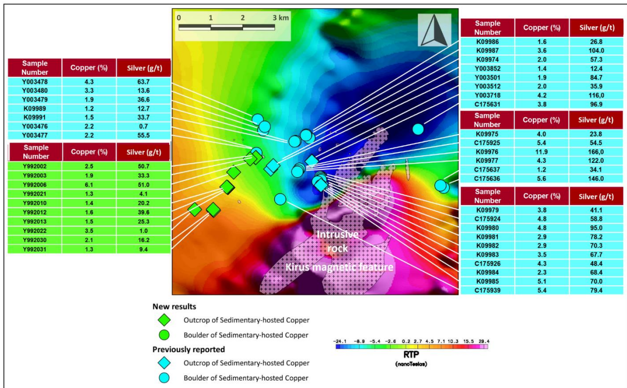
Abbildung 1. Lage der hochgradigen Kupfer-Silber-Proben, die aus Aufschlüssen und Felsblöcken in Flüssen im Zielgebiet Kirus entnommen wurden. Dargestellt über den Magnetik-Daten (negative Reduktion zum Äquator, was in etwa der Reduktion zum Pol („RTP“) entspricht).
