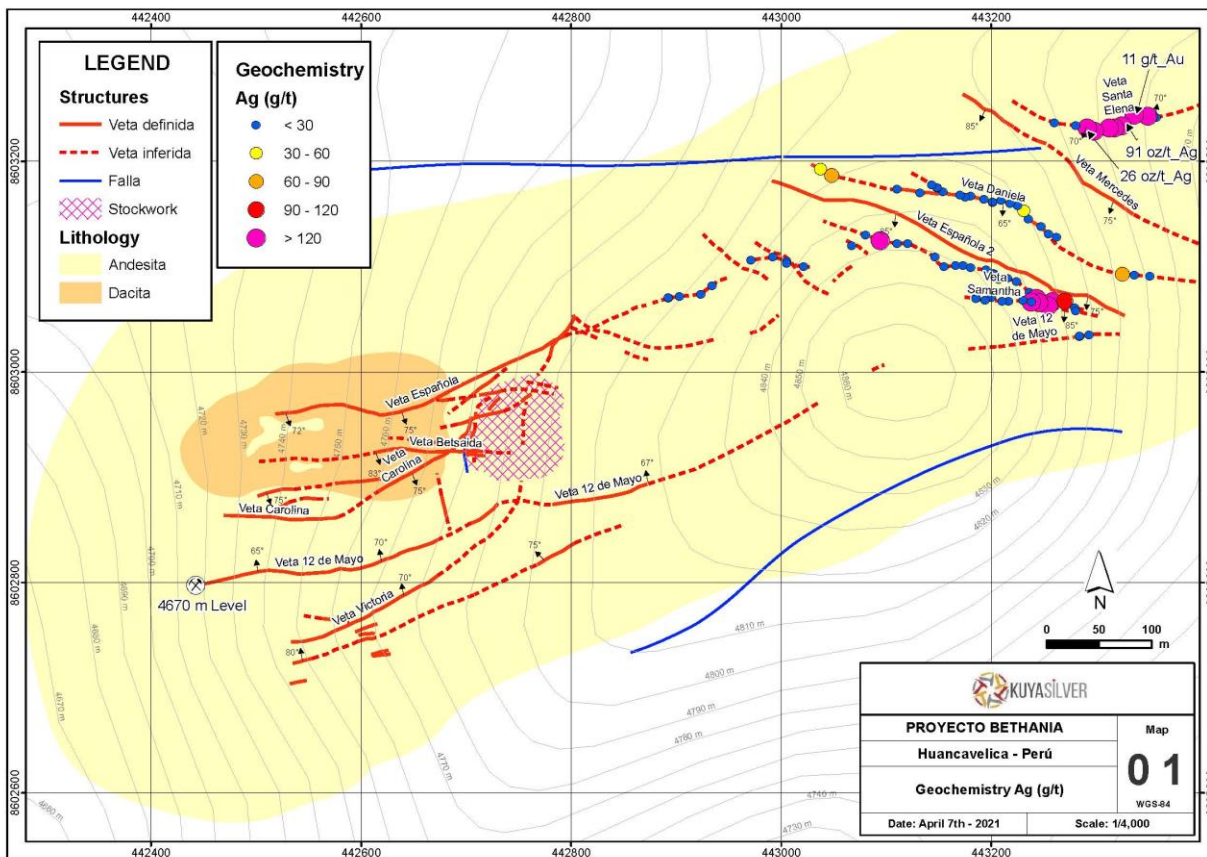
Abb. 1: Geochemie-Karte mit Lage und Ergebnisse der Gesteinssplinterproben auf dem Projekt Bethania
